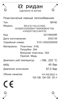
Рис.5 – Пример шильда пластинчатого паяного теплообменника ВРНЕ
