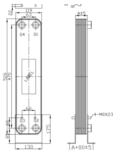
Рис.6 - Габаритные размеры и изображение теплообменника пластинчатого модификации BPHE_RD-060
